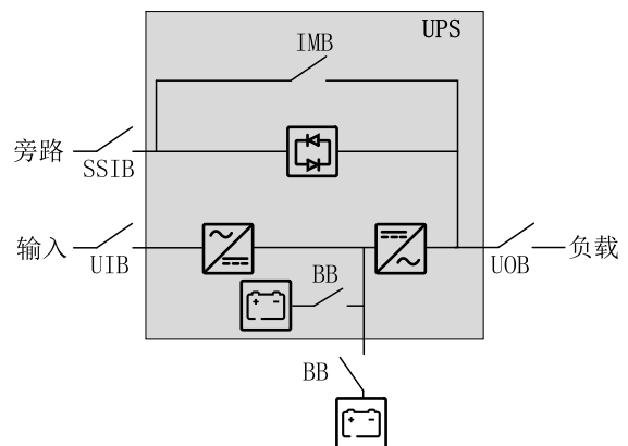
单机系统 - 双市电
