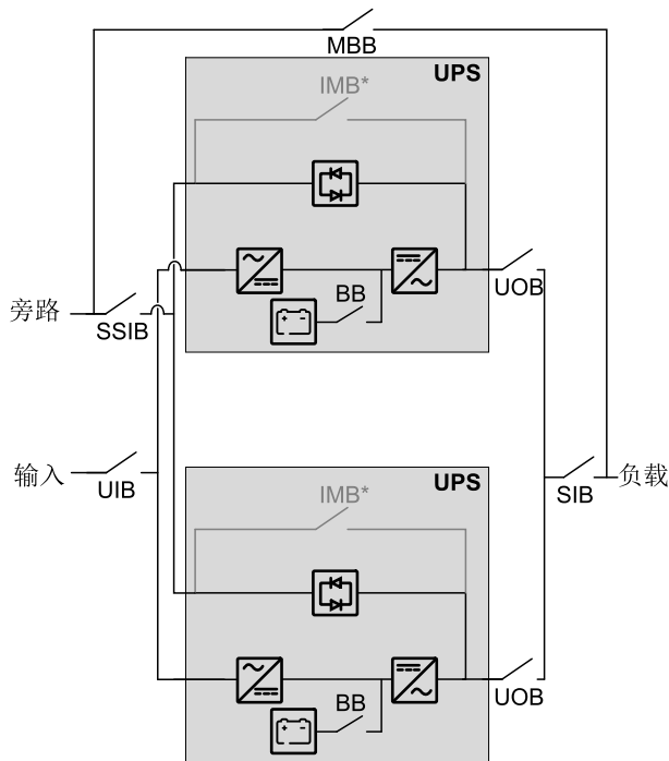
并机系统 - 双市电
