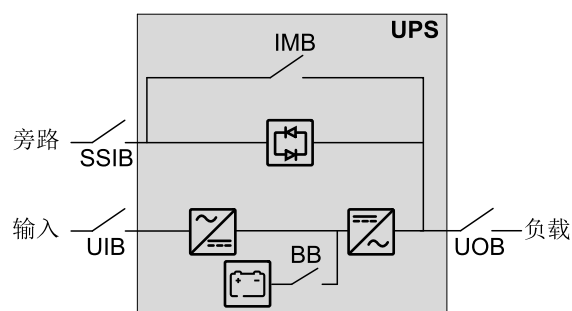
单机系统 - 双市电
