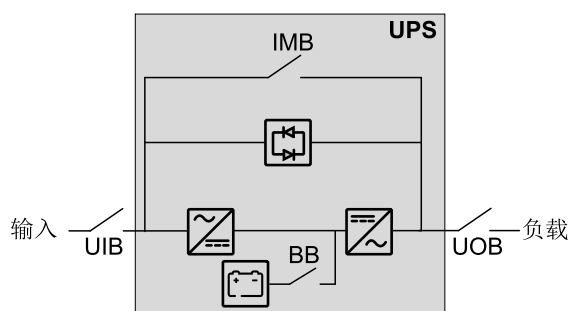
单机系统 - 单市电
